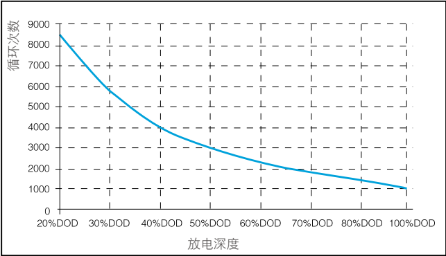
不同放电深度下的循环曲线
