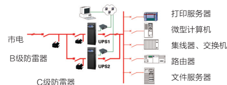
双机并联拓扑图
